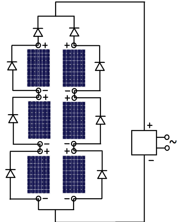
Vereinfachtes Schaltbild einer Solaranlage
